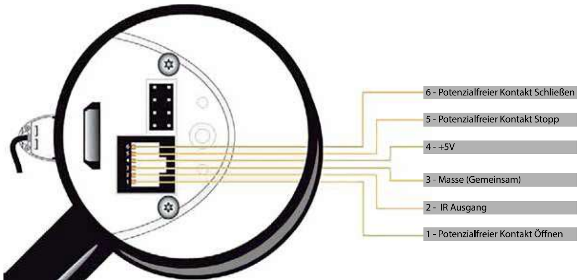
Anschlussbeispiel
